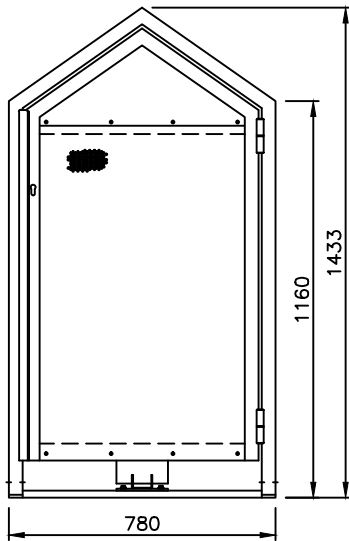
vooraanzicht
